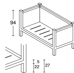
Struttura smontabile
