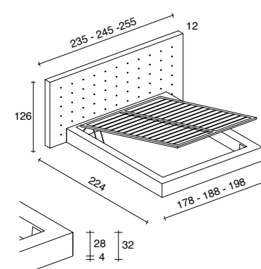
Struttura smontabile
