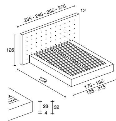
Base Smontata
