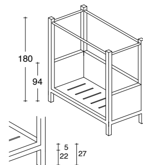
Struttura smontabile
