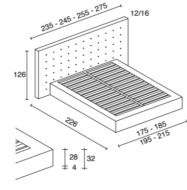
Base Smontata
