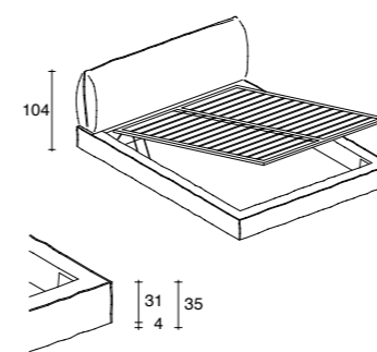
Struttura smontabile
