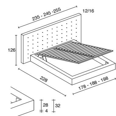
Struttura smontabile
